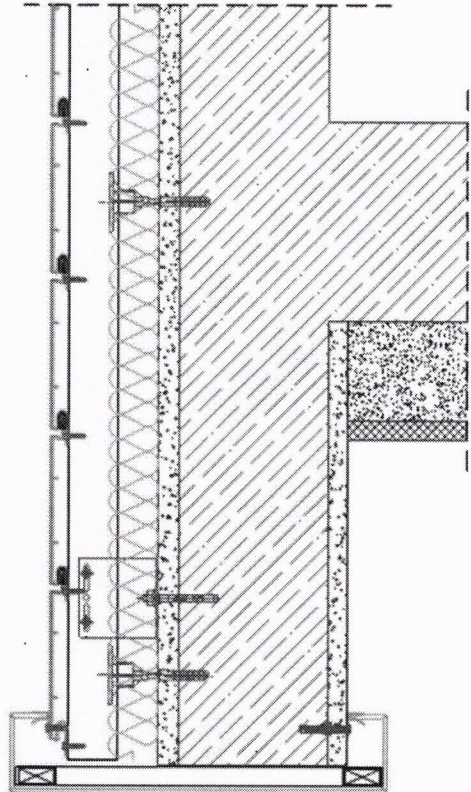
12 PARAPET DETAYI 1
