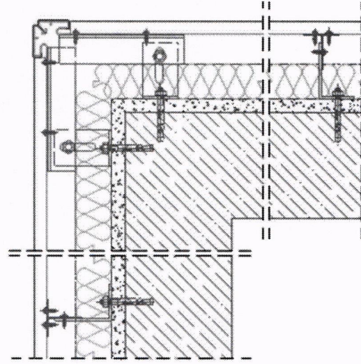
② KÖŞE DÖNÜŞ DETAYI 2
