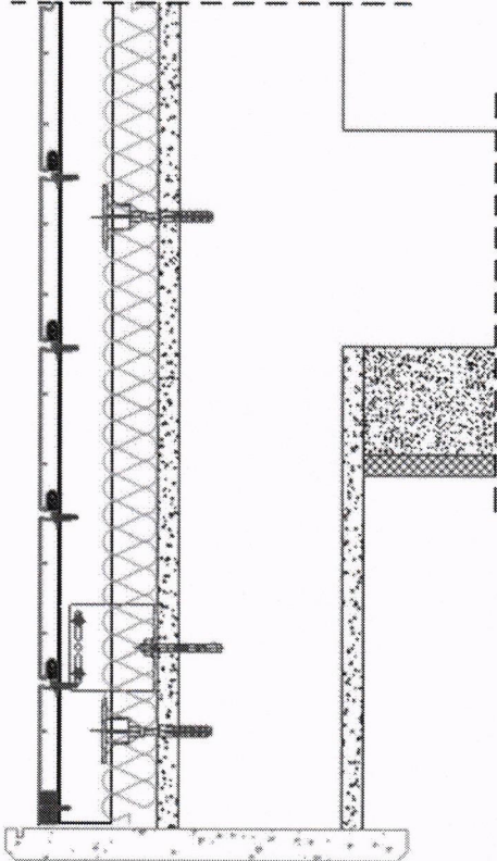
13 PARAPET DETAYI 2
