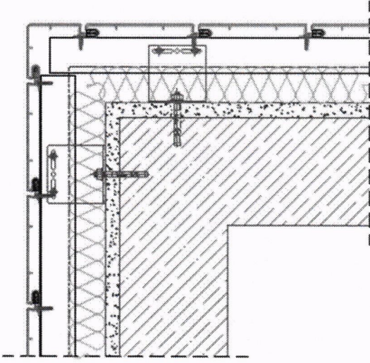
11 DİKEY DÖŞEME KÖŞE DÖNÜŞ
