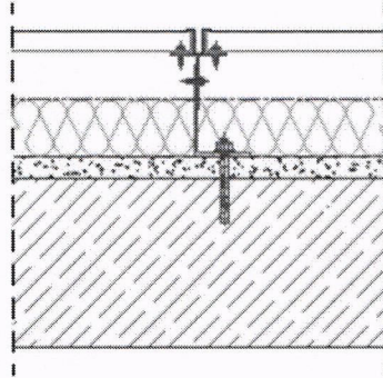
④ BİRLEŞİM DETAYI 2
