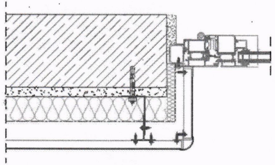
14 DOĞRAMA DÖNÜŞ DETAYI 1
