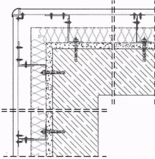
① KÖŞE DÖNÜŞ DETAYI 1
