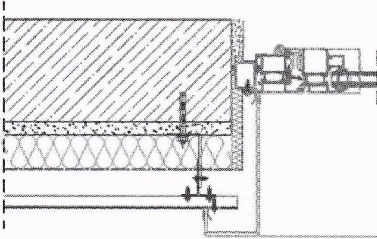
15 DOĞRAMA DÖNÜŞ DETAYI 2
