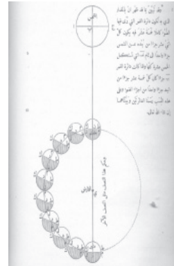
Zic-i Sâbi'de Ay'ın evreleri
